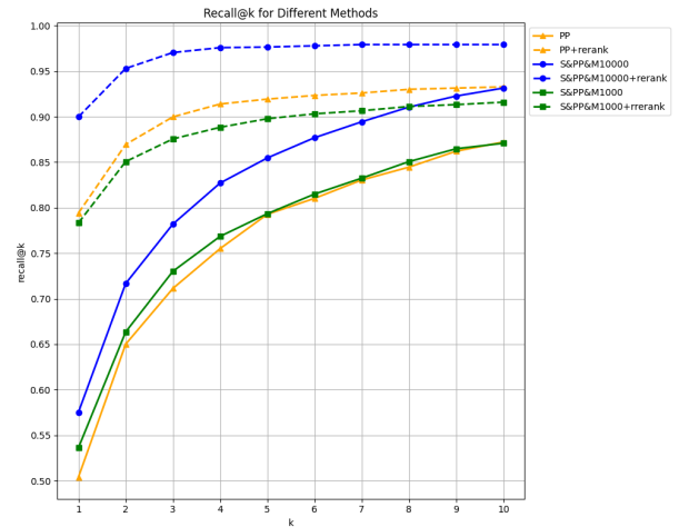
FIGURE 2 – Comparaison des résultats sur le retriever avec et sans reranking . En ligne pleine les résultats avec un RAG classique et en pointillé avec un RAG augmenté par reranking
